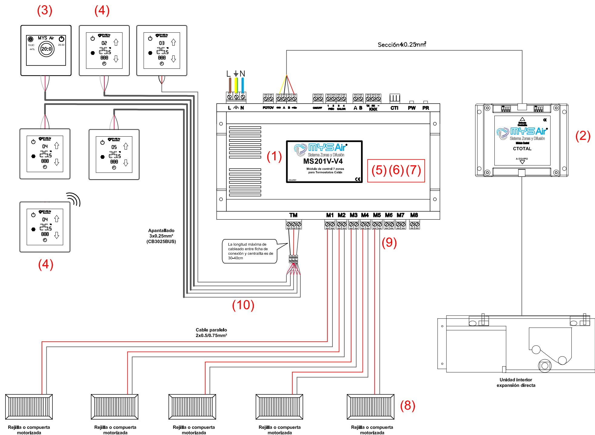
DETALLE TIPOLOGÍA DE MÓDULOS DE CONTROL (MONTAJE DENTRO DE CENTRAL)
