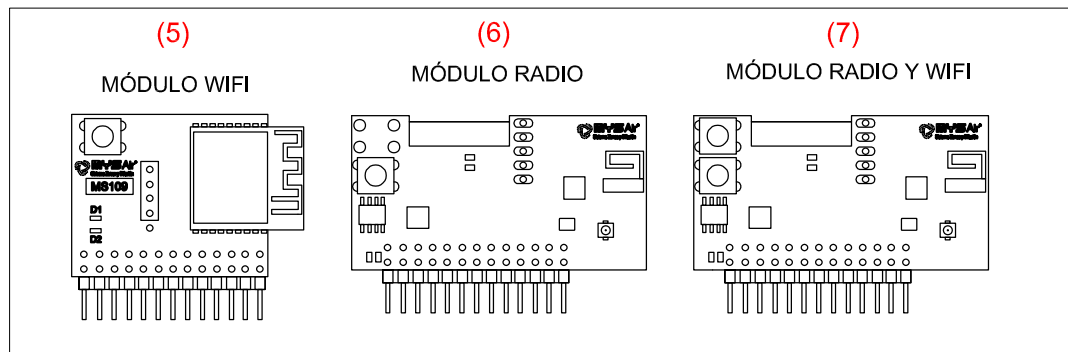
DETALLE TIPOLOGÍA DE MÓDULOS DE CONTROL (MONTAJE DENTRO DE CENTRAL)
